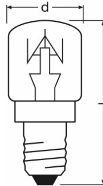
SPC.T OVEN CL 15 W 230 V E14, SPC.T OVEN CL 15 W 240 V E14
