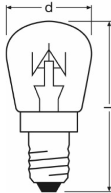
SPC.T CL 15 W 230 V E14, SPC.T CL 25 W 250 V E14
