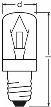
SPC.T CL 15 W 230 V E14
